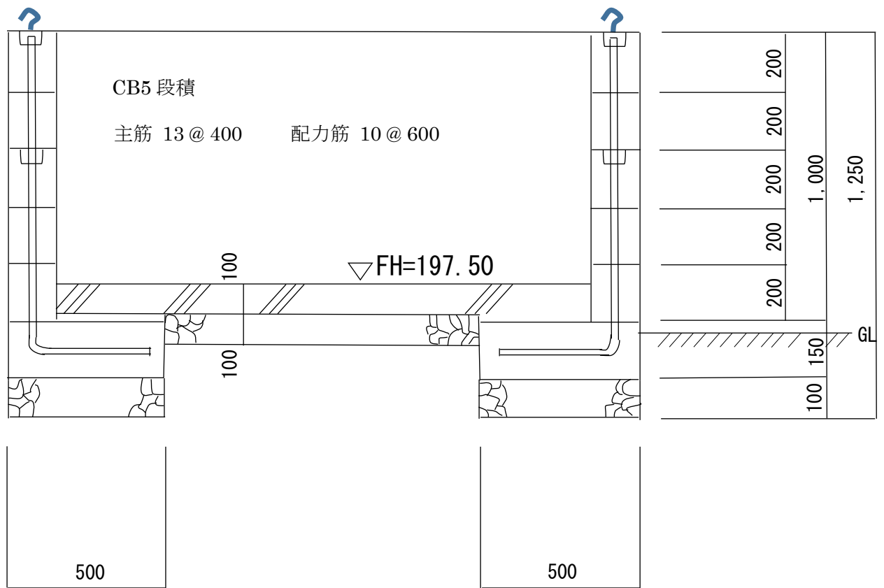
X ゴミ収集場所断面図 S=1/30
