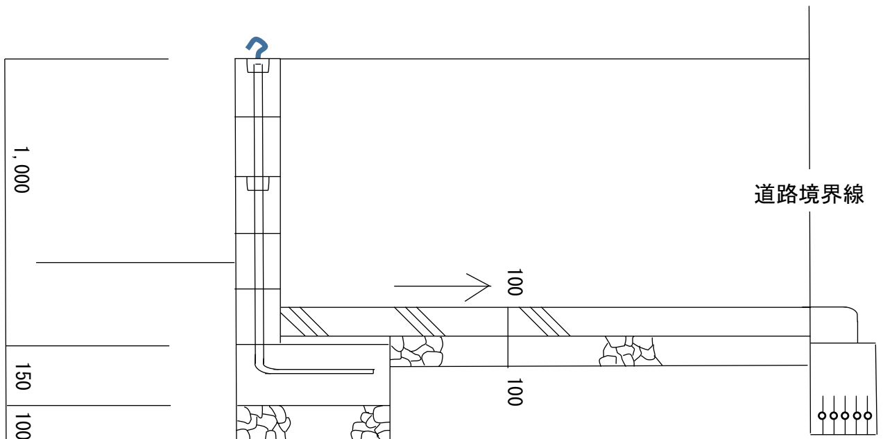
X ゴミ収集場所断面図 S=1/30
